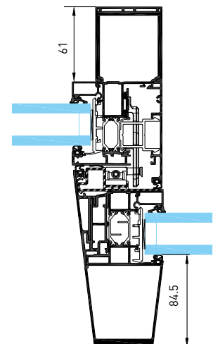
Horizontal sektion – förstärkt möteslösning
