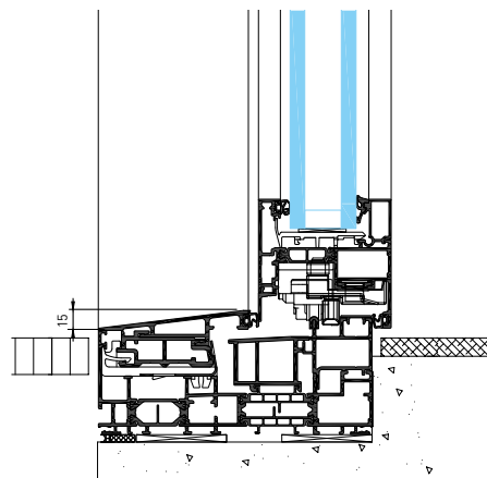
Vertikal sektion – dörrblad, låg tröskel
