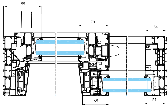
Horizontal sektion – 1 dörrblad + fast parti
