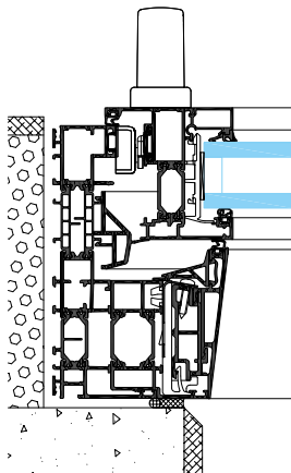
Horizontal sektion – inbyggt dörrblad
