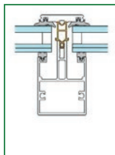
2-lags isolerglass
