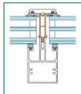
3-lags isolerglass
