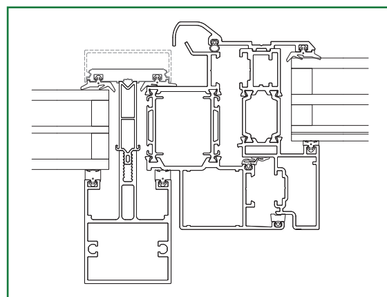
Luke, 2- eller 3-lags isolerglass
